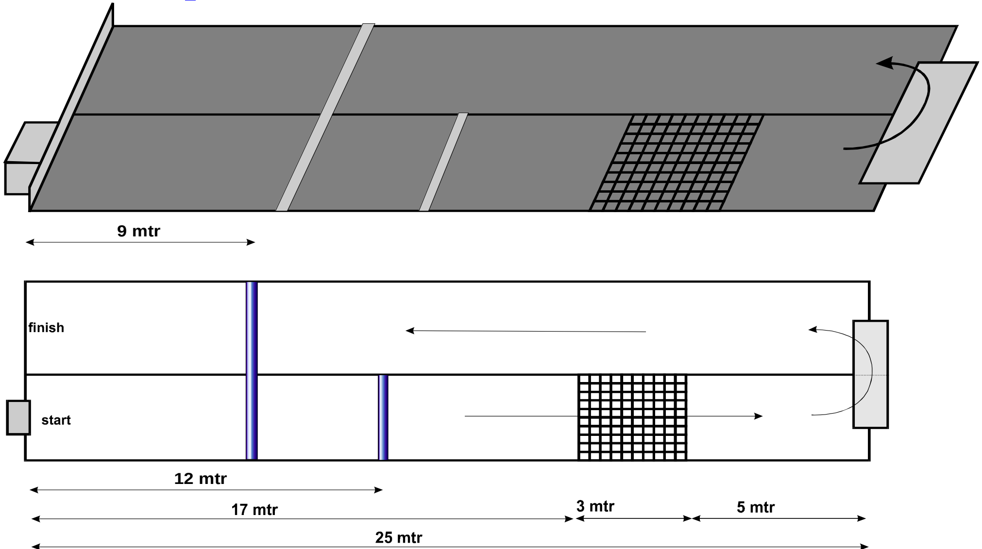
SITUATIETEKENING 25M BAD ↑
